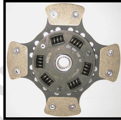
Sinterplaat
